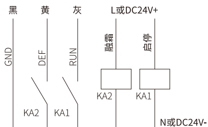
图 5 有源输入接法
